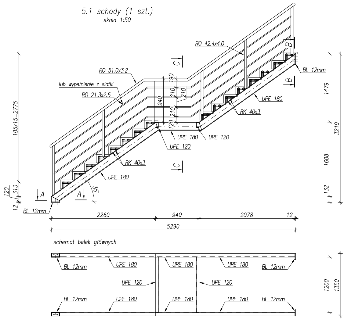
stopnie betonowe gr.40mm 260x1350mm 17 szt
